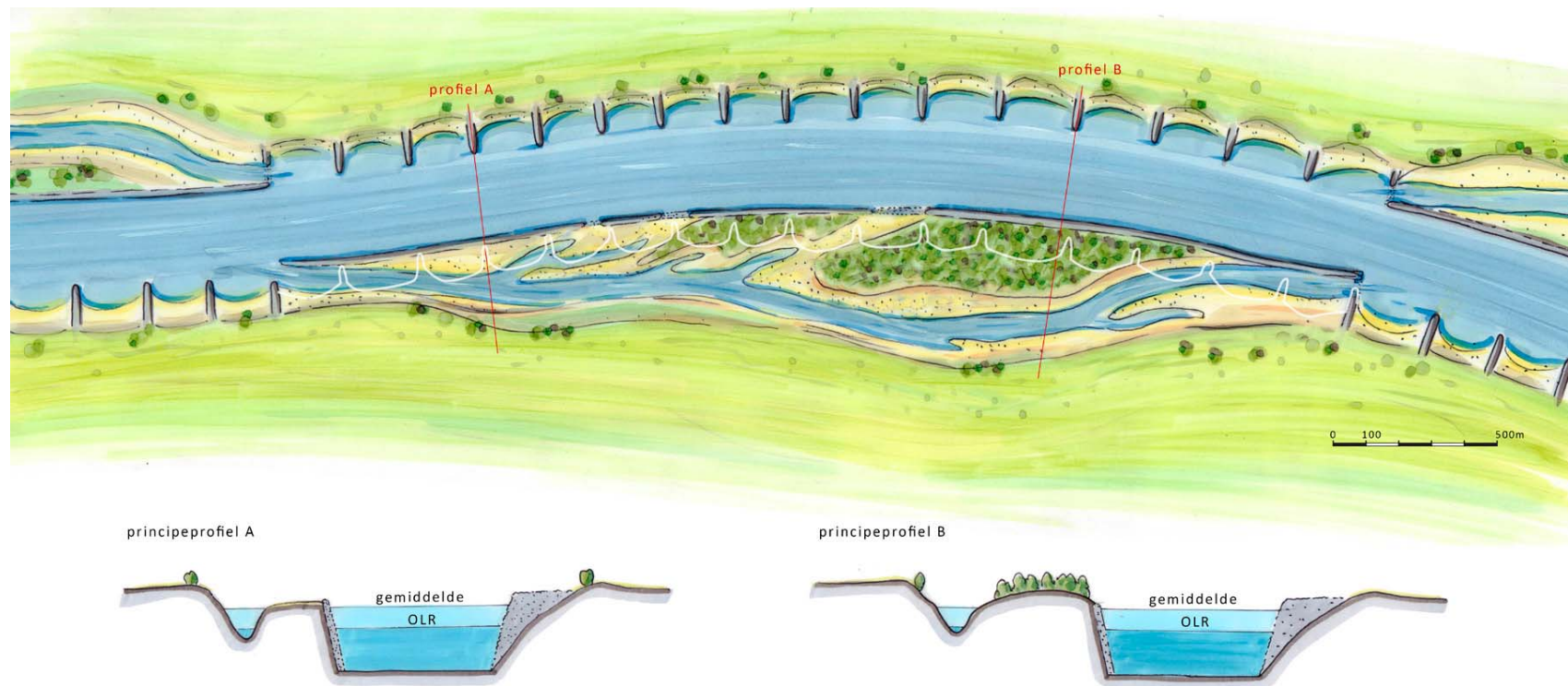
Principeontwerp van meestromende nevengeulen langs de Middenwaal (2020)
